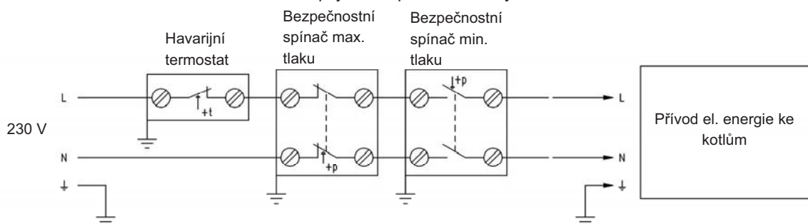
Elektrické zapojení bezpečnostní sady INAIL
