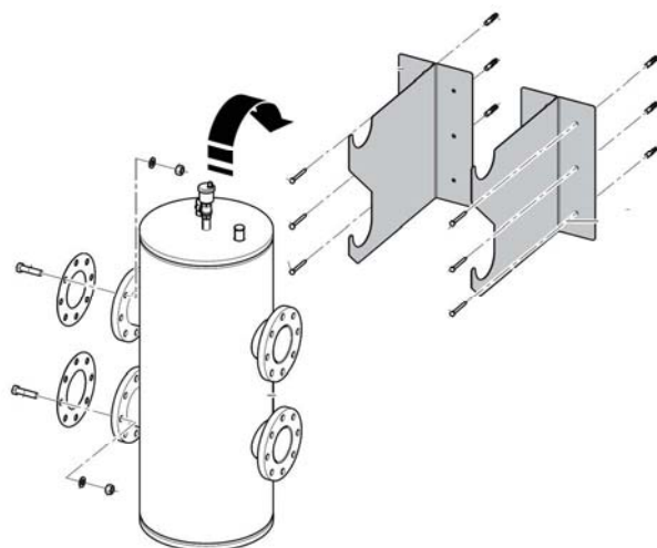
Držák na stěnu
