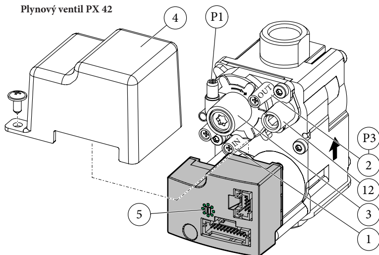
Plynový ventil PX 42
