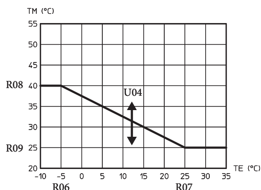
Teplota na prívode do miešanej zóny 2 počas ohrevu s nainštalovanou vonkajšou sondou
