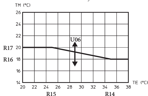
Teplota na prívode počas chladenia bez vonkajšej sondy
